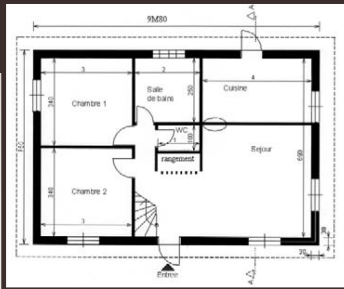
◀ Plan rez-de-chaussée
