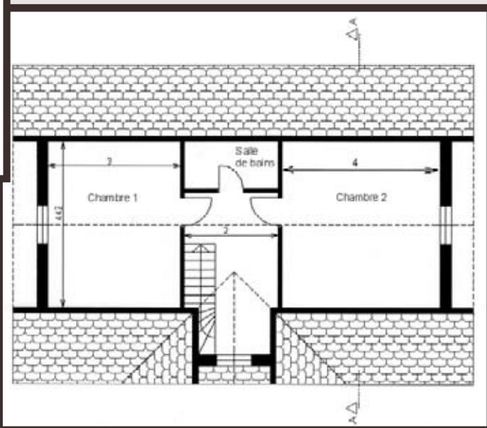
▼ Plan étage
