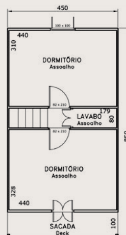
PAVIMENTO SUPERIOR A: 38,25 M2
